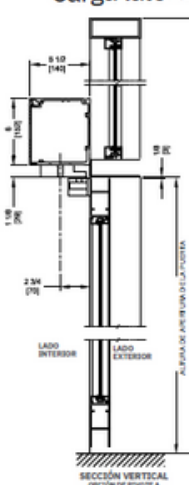
GT8400 Carga lateral
