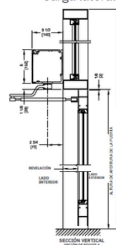
GT8400 Carga lateral
