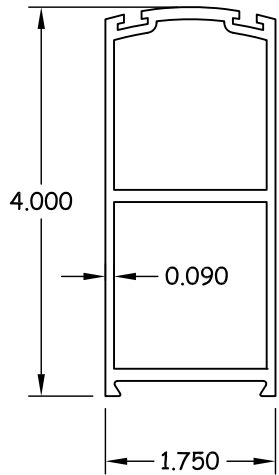
5 4" STILE 6063-T6
