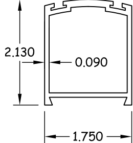
12 STILE 6063-T6
