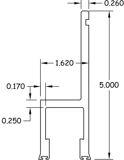
7 DOOR CARRIER 6063-T6
