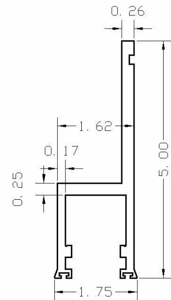
14-9015 INTERFACE LEG ALLOY: 6063-T5
