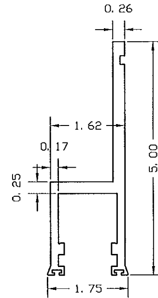
14-9015 INTERFACE LEG ALLOY: 6063-T5
