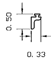
14-9015 INTERFACE LEG ALLOY: 6063-T5
