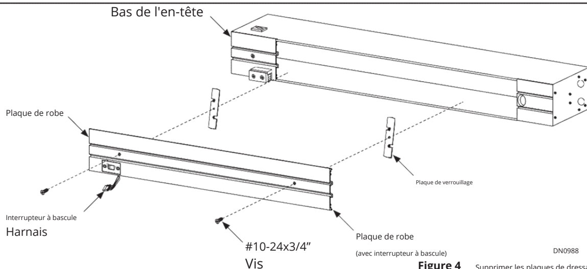
DN0988 Figure 4 Supprimer les plaques de dressage de l'en-tête
