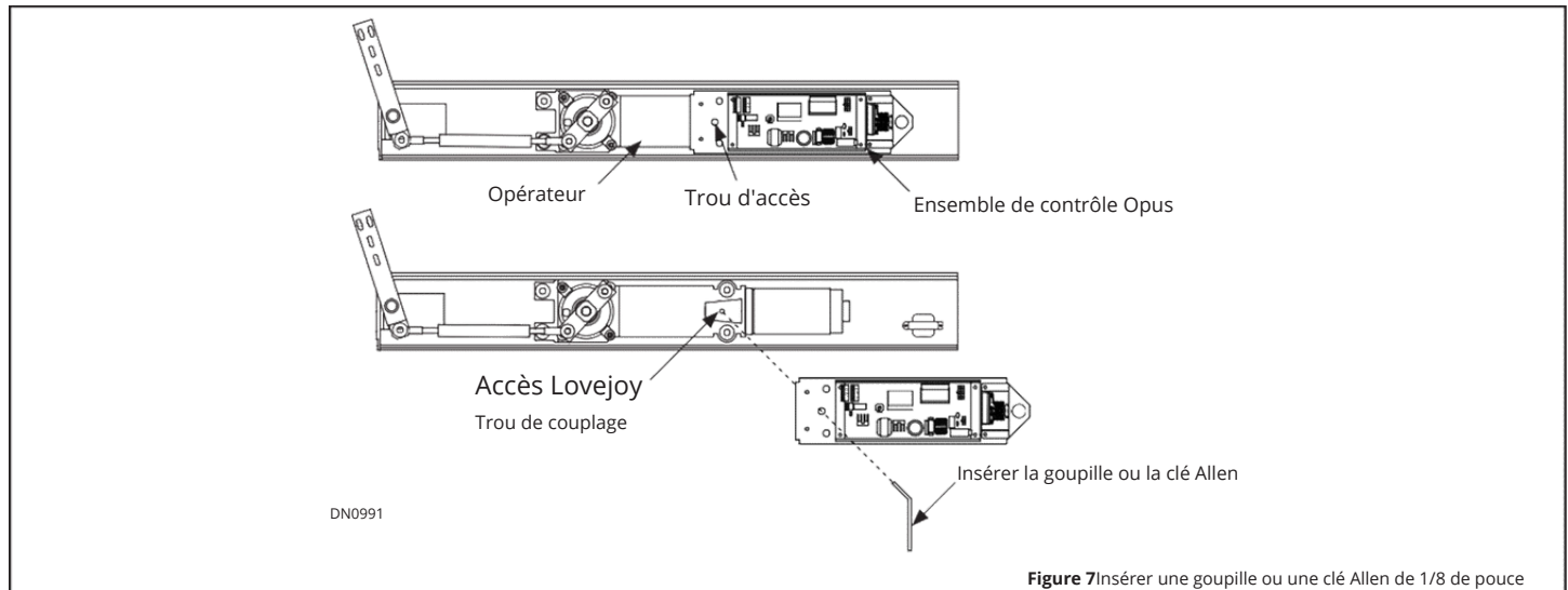
Figure 7 Insérer une goupille ou une clé Allen de 1/8 de pouce
