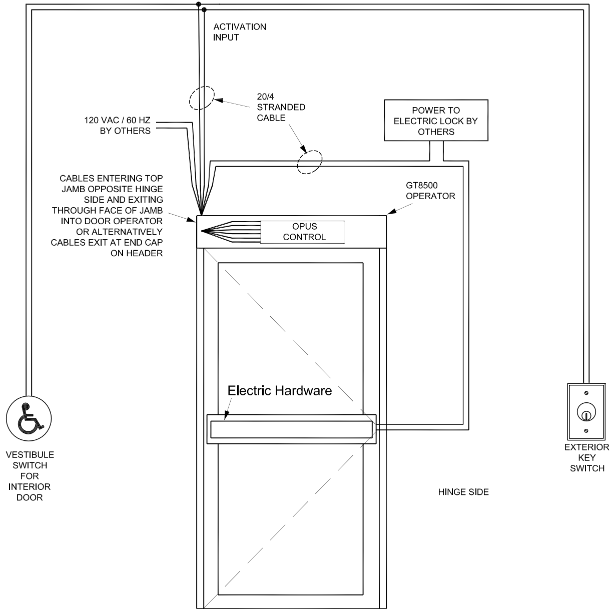
GT8500 DOOR RISER DIAGRAM
