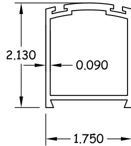
12 STILE 6063-T6
