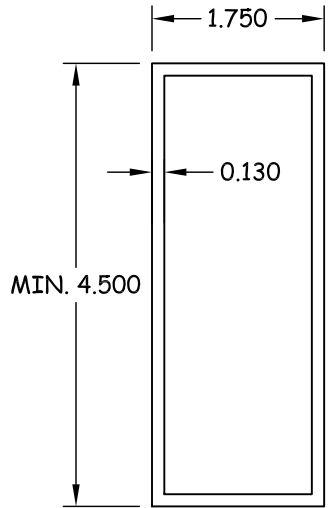
10 JAMB EXT. 6063-T5
