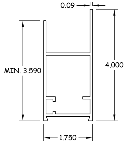
16 TOP RAIL DOOR 6063-T6
