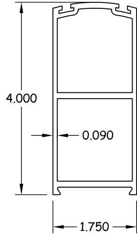
5 4" STILE 6063-T6
