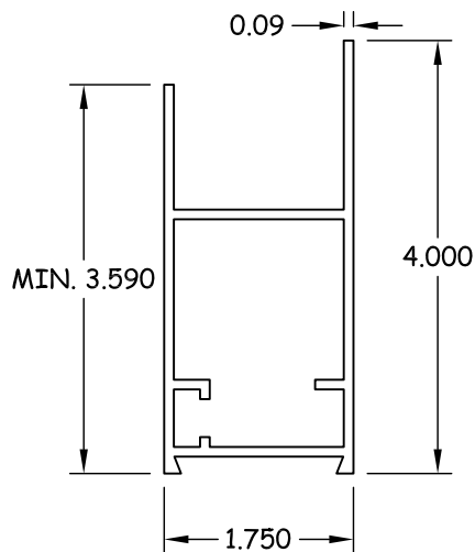
16 TOP RAIL DOOR 6063-T6
