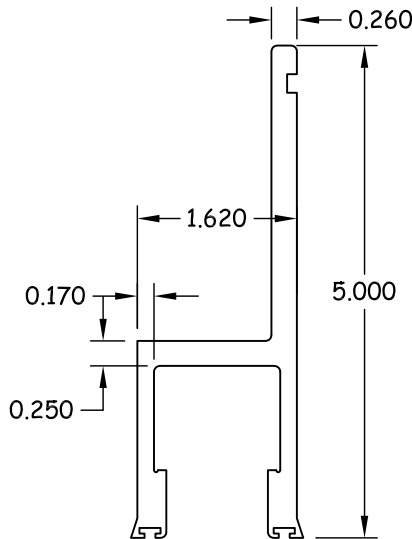
7 DOOR CARRIER 6063-T6
