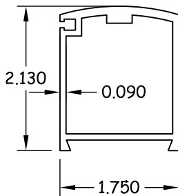
11 2" PIVOT STYLE 6063-T6
