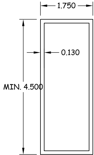
10 JAMB EXT. 6063-T5
