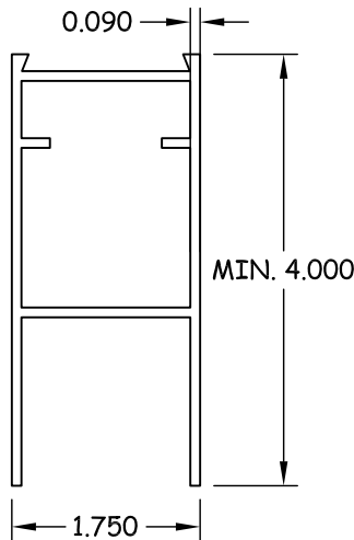
17 BOTTOM RAIL DOOR 6063-T6
