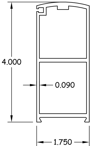
4 4" PIVOT STILE 6063-T6
